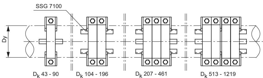
Figuren gäller båda klammerhalvorna
